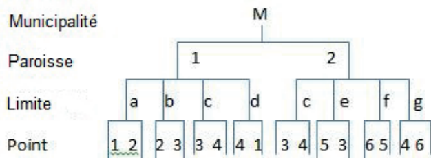
Figure 3.4 : La structure hiérarchique des deux paroisses de la figure 3.3. On voit que le segment « c » figure deux fois, et que tous les points figurent deux fois, sauf les points 3 et 4, qui figurent 4 fois.
